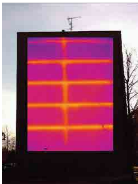
UDINE - EDILIZIA ECONOMICA POPOLARE, ANNI '70 IN EVIDENZA LE DISPERSIONI TERMICHE CORRISPONDENTI ALLE STRUTTURE PORTANTI
