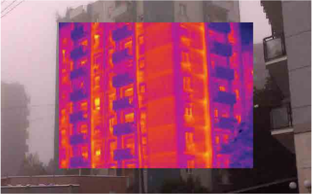
MILANO - VIA PADOVA, EDILIZIA RESIDENZIALE PRIVATA, ANNI '70 >>
